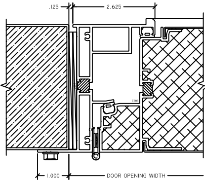
1 HINGE JAMB SD4200 NEG
