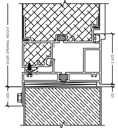
4 SILL SD4200 NEG
