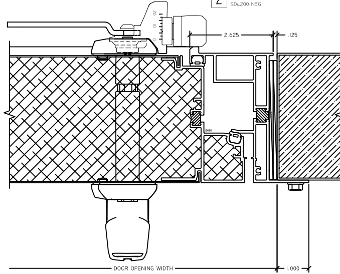
2 LOCK JAMB SD4200 NEG
