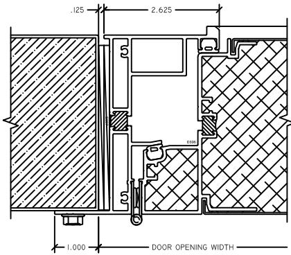
1 HINGE JAMB SD4200 NEG
