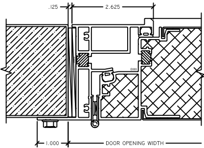
1 HINGE JAMB SD3200 NEG
