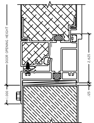
4 SILL SD3200 NEG
