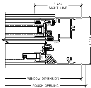
4 OP JAMB Z560 SH
