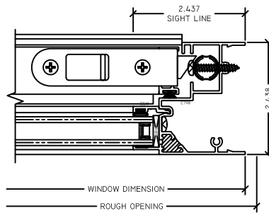
2 FX JAMB S260 SH
