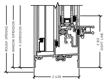
7 SILL S260 SH
