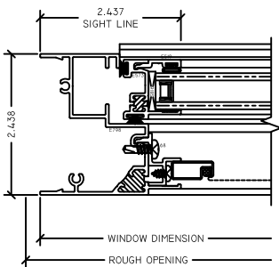
3 OP JAMB Z560 SH
