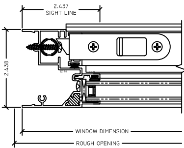
1 FX JAMB S260 SH
