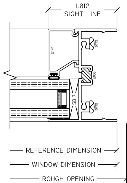
6 FX JAMB S220 FXD
