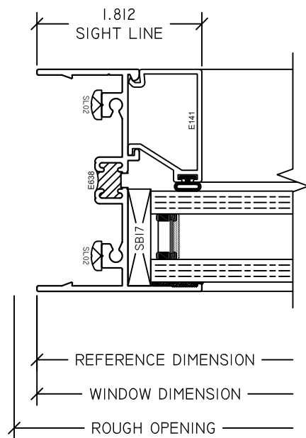
4 FX JAMB S220 FXD
