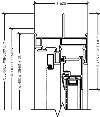
1 OP HEAD RV STANDARD FIN SLIDER
