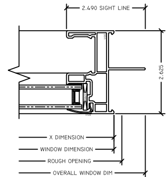
7 FX JAMB RV STANDARD FIN SLIDER
