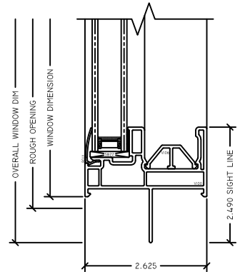
4 FX SILL RV STANDARD FIN SLIDER
