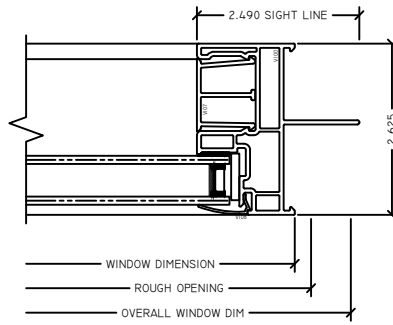
④ RJAMB RV STANDARD FIN FX
