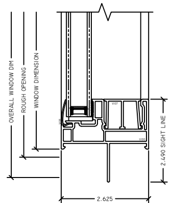
② SILL RV STANDARD FIN FX
