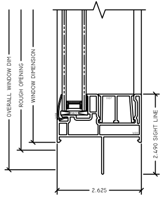
2 SILL RV STANDARD FIN FX
