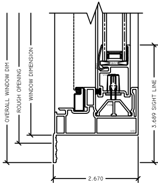
2 OP SILL RV OUTSIDE FIN SLIDER
