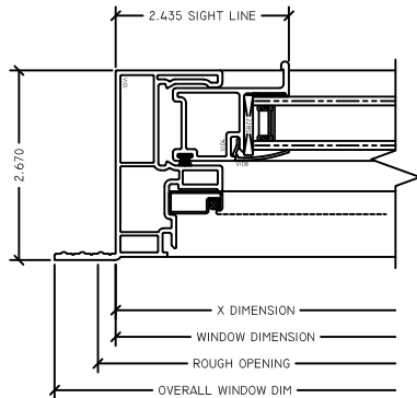
5 OP JAMB RV OUTSIDE FIN SLIDER
