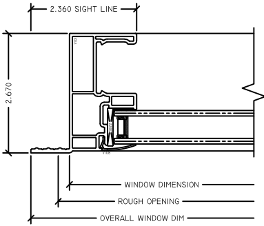
4 FX LJAMB RV OUTSIDE FIN SH
