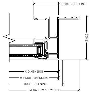
7 FX JAMB RV INSIDE FIN SLIDER
