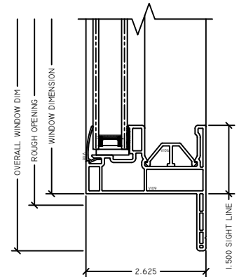
4 FX SILL RV INSIDE FIN SLIDER
