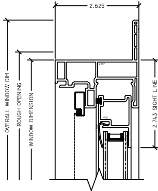
1 OP HEAD RV INSIDE FIN SLIDER
