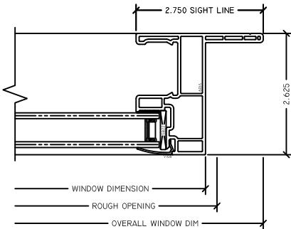
5 FX RJAMB RV INSIDE FIN SH
