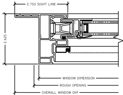
6 OP LJAMB RV INSIDE FIN SH
