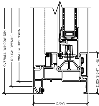
2 OP SILL RV BOMAN SLIDER
