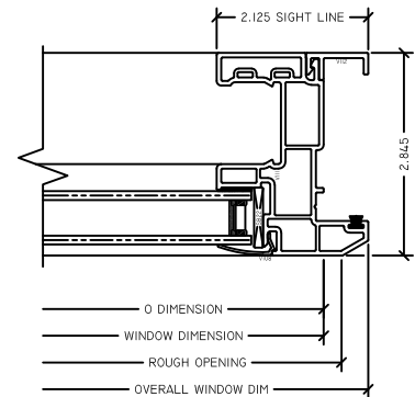
7 FX JAMB RV BOMAN SLIDER
