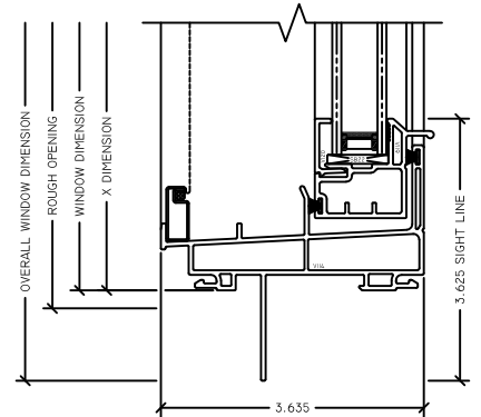
2 SILL OVDH
