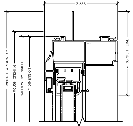
1 HEAD OVDH
