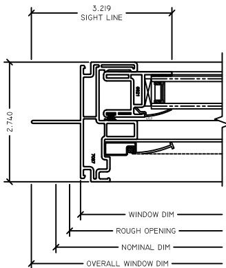
5 OP LJAMB MB70 SLIDER
