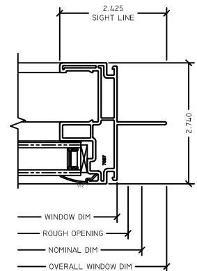
7 FX LJAMB MB70 SLIDER
