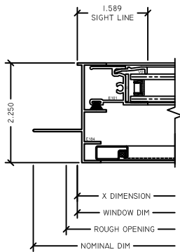
5 OP LJAMB M225 SLIDER
