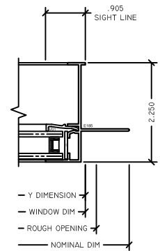
7 FX RJAMB M225 SLIDER
