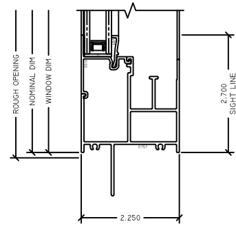
4 FX SILL M225 SLIDER
