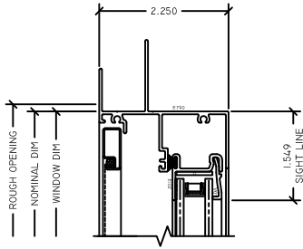
1 OP HEAD M225 SLIDER
