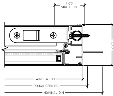
2 FX JAMB M225 SH
