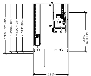
7 SILL M225 SH
