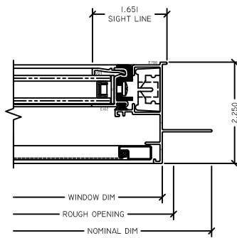
4 OP JAMB M225 SH
