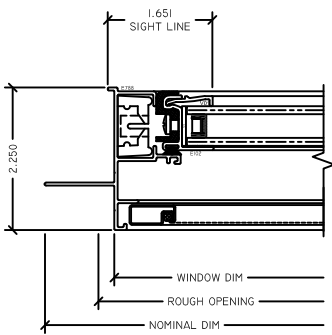
3 OP JAMB M225 SH
