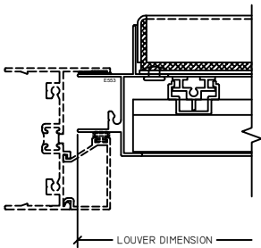
5 JAMB H2211 BLANK OFF
