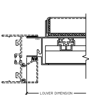
5 JAMB H221 BLANKOFF
