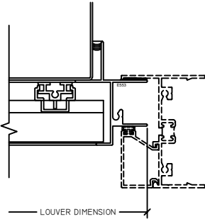
2 JAMB H221
