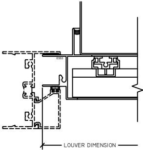
1 JAMB H221
