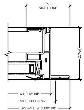
7 FXRJAMB G75/G78 SLIDER
