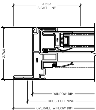
5 OPLJAMB G75/G78 SLIDER
