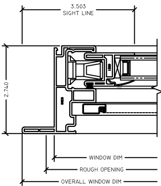
6 OP LJAMB G75/G78 SH
