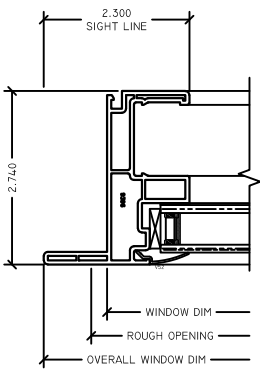
4 FX LJAMB G75/G78 SH
