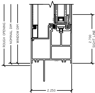
2 OP SILL G225 SLIDER
