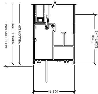
4 FX SILL G225 SLIDER
