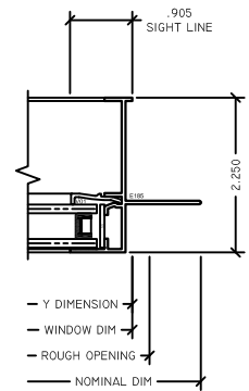
7 FX RJAMB G225 SLIDER
