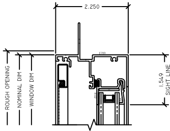
1 OP HEAD G225 SLIDER
