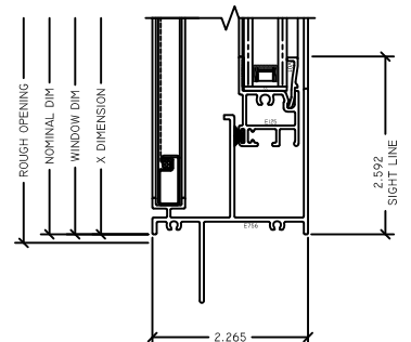
7 SILL G225 SH
