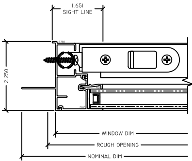
1 FX JAMB G225 SH
