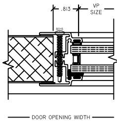
7 VP JAMB ADI500 POS
