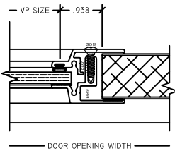
8 VP JAMB AD1100 POS
