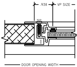
7 VP JAMB AD1100 POS
