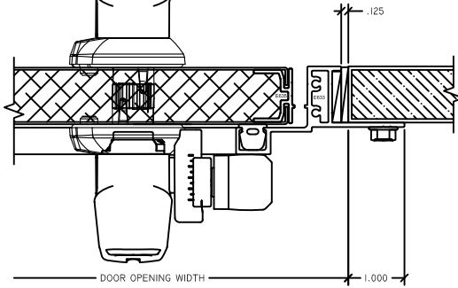
2 LOCK JAMB AD1100 POS
