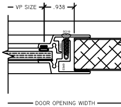
8 VP JAMB AD1100 NEG
