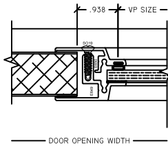
7 VP JAMB AD1100 NEG
