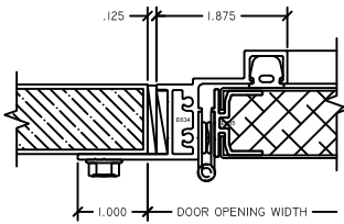
1 HINGE JAMB AD1100 NEG
