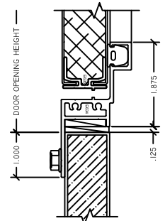
6 SILL AD1100 NEG
