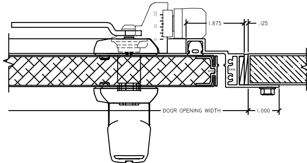
2 LOCK JAMB AD1100 NEG
