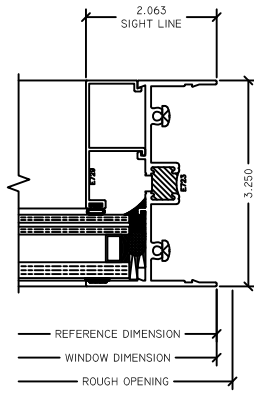
5 FX RJAMB 3501 FX
