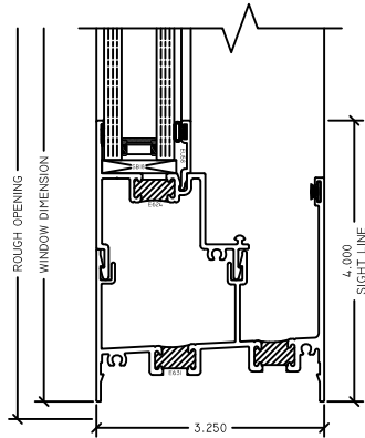
3 FX SILL 3210 HS
