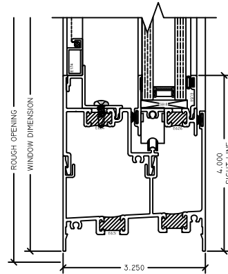
4 OP SILL 3210 HS
