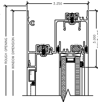
2 OP HEAD 3210 HS
