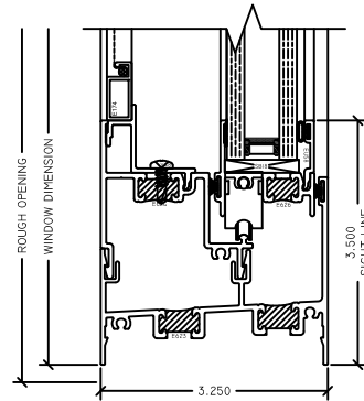
4 OP SILL 3210 HS
