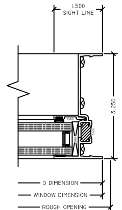
8 FX JAMB 3210 HS
