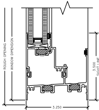
3 FX SILL 3210 HS
