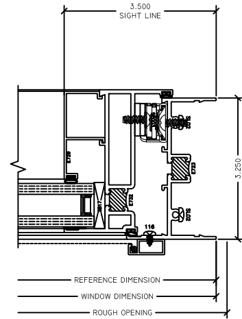
4 PI RIGHT JAMB 320 PI
