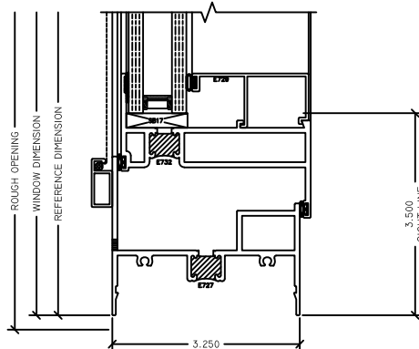
2 PI SILL 320 PI
