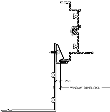
3 SQ. PANNING LEFT JAMB
