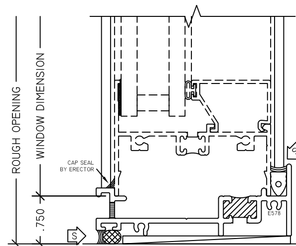
4 SILL SUBFRAME
