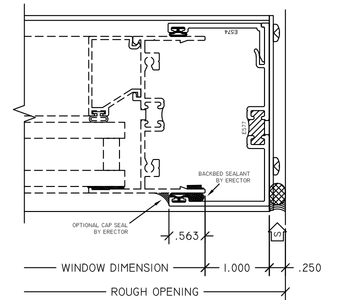
2 JAMB SUBFRAME
