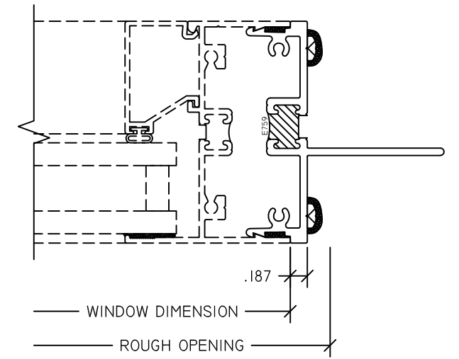
2 JAMB NAIL FIN
