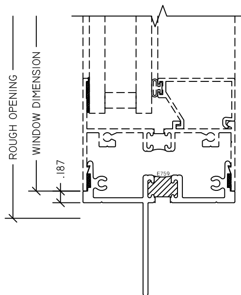
4 SILL NAIL FIN
