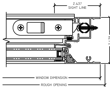
2 FX JAMB 2560 SH
