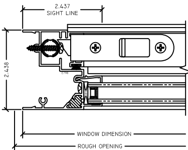
1 FX JAMB 2560 SH
