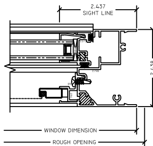
4 OP JAMB 2560 SH
