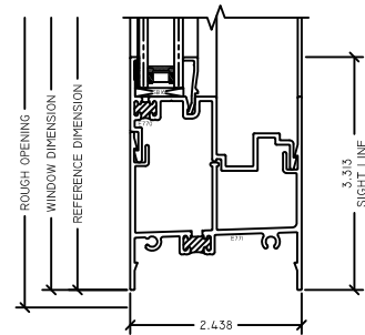
4 FX SILL 2510 SLIDER
