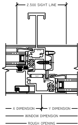
6 XO MTG. RAIL 2510 SLIDER
