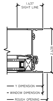
7 FX JAMB 2510 SLIDER
