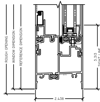
4 OP SILL 2510 SLIDER
