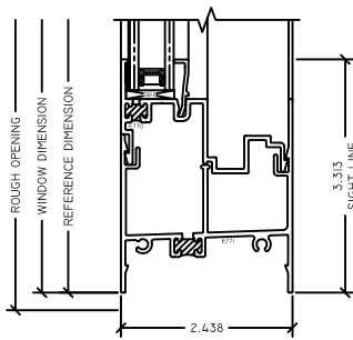
3 FX SILL 2510 SLIDER
