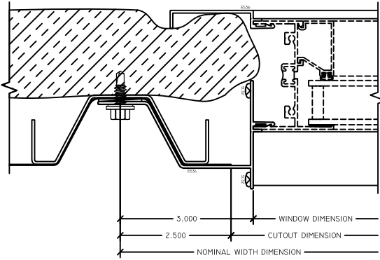
1 JAMB SHADOWWALL FIN
