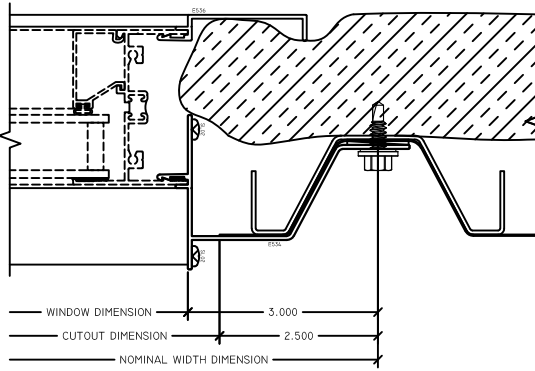
2 JAMB SHADOWWALL FIN
