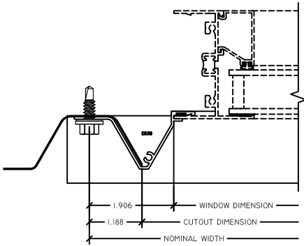
1 JAMB ARCHITECTURAL FIN
