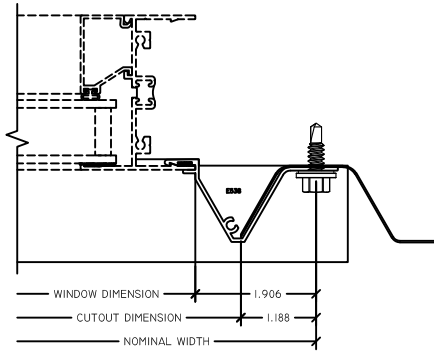
2 JAMB ARCHITECTURAL FIN
