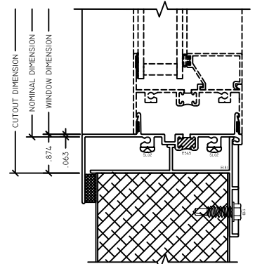
4 SILL 3" INSULVIEW FIN
