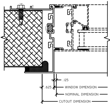
1 JAMB 3" INSULVIEW FIN
