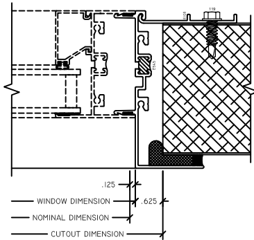
2 JAMB 3" INSULVIEW FIN
