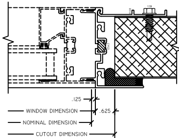
2 JAMB 2" INSULVIEW FIN
