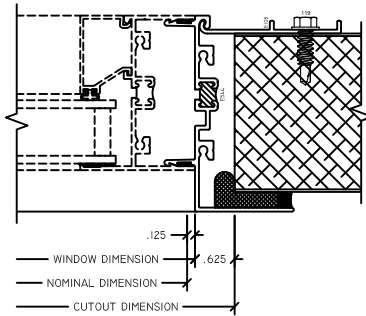
2 JAMB 2-1/2" INSULVIEW FIN
