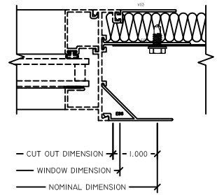
4 JAMB 225 STRAIGHT JAMB FIN
