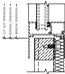
2 SILL 225 STRAIGHT JAMB FIN
