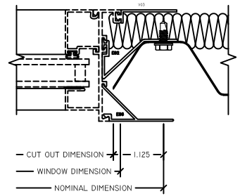
4 JAMB 225 ARCHITECTURAL FIN
