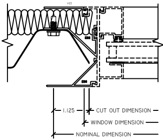
3 JAMB 225 ARCHITECTURAL FIN
