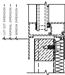
2 SILL 225 ARCHITECTURAL FIN
