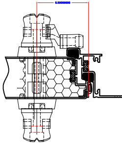
1 1/2" - 2" DOOR 2 GASKET
