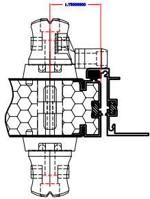
1 1/2" - 2" DOOR 1 GASKET
