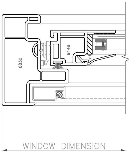
3 LEFT JAMB SERIES 70 V200 PI HOPPER
