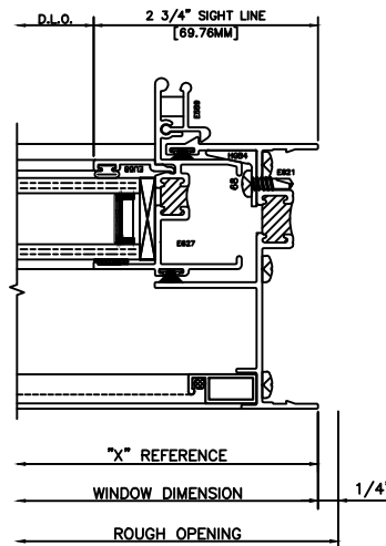
52 SASH JAMB 3210 SLIDER
