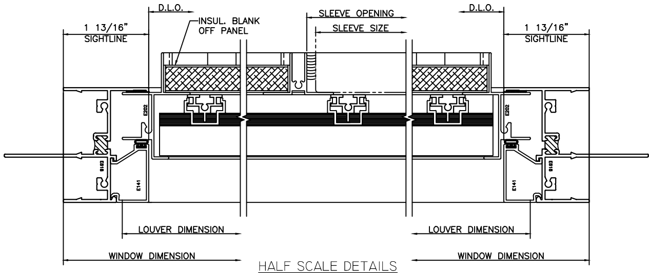
21 LOUVER JAMB
