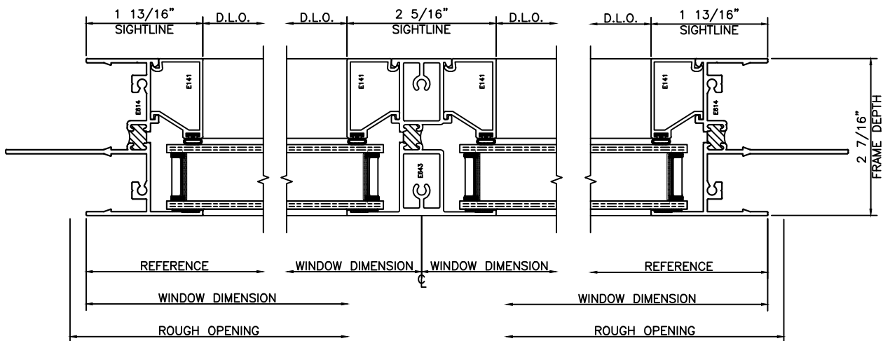
4 FIXED JAMB
