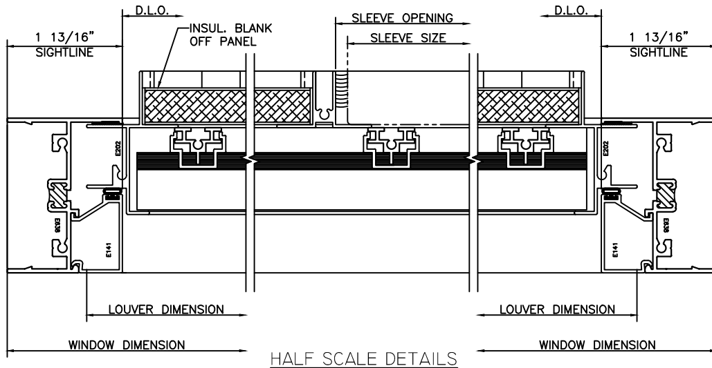
21 LOUVER JAMB
