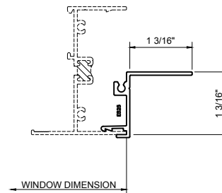
E525 ALUMINUM NAIL FIN
