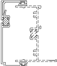
E160 SUBFRAME
